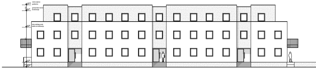
SHEMATSKI PRIKAZ: SJEVERNO PROČELJE
