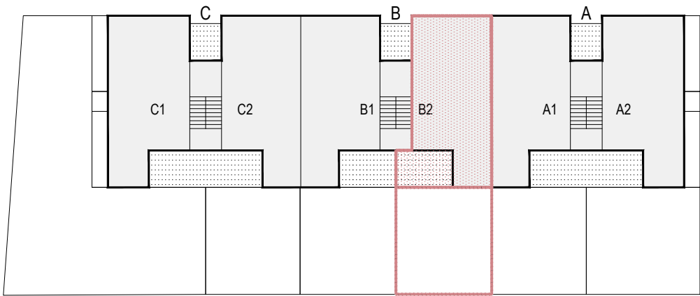
SHEMATSKI PRIKAZ: TLOCRT PRIZEMLJA
